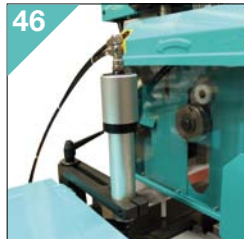
46 691100 - SIRIO Etiau verticale pneumatique. / Mordaza vertical neumatica.
