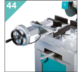
44 PERFECT 300 - RECORD - SIRIO Etiau pneumatique. Mordaza neumatica.
