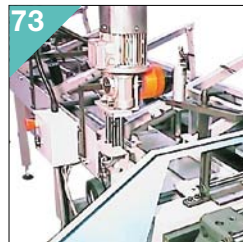
73 000935-01 SIRIO 370 AF-NC SLB6 VELOX 350 AF-NC SLB6 Guides supérieurs pour diamètres jusqu'à 10mm. Guías superiores para diámetros inferiores a 10mm.
