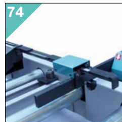
74 RL RTR Butée de mesure digitale avec recul automatique. Lector de medida digital y ralentizador automático.
