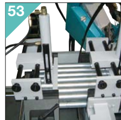
53 AUTOMATICQUES SERIE BS - AUTOMATICAS BS SERIES Dispositif hydraulique coupe en paquet. Aparato hydraulico para corte a paquete.
