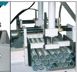
53 AUTOMATICQUES SERIE BS - AUTOMATICAS BS SERIES Dispositif hydraulique coupe en paquet. Aparato hydraulico para corte a paquete.
